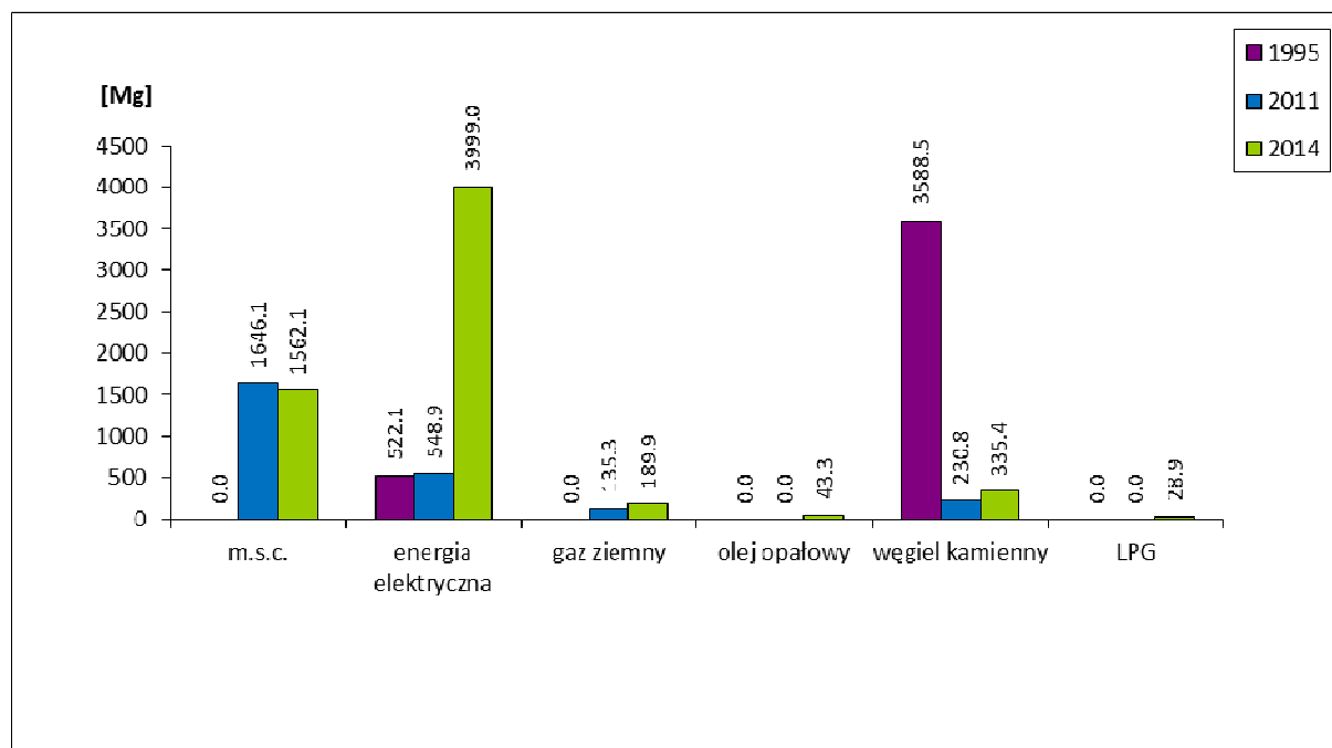
Rysunek 4. Emisja CO 2 - obiekty użyteczności publicznej.
