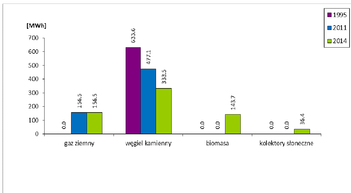
Rysunek 6. Końcowe zużycie energii - budynki mieszkalne komunalne.
