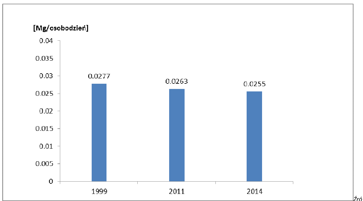
Rysunek 26. Emisja CO 2 na jeden osobodzień (mieszkańcy oraz turyści) z pominięciem przemysłu.
