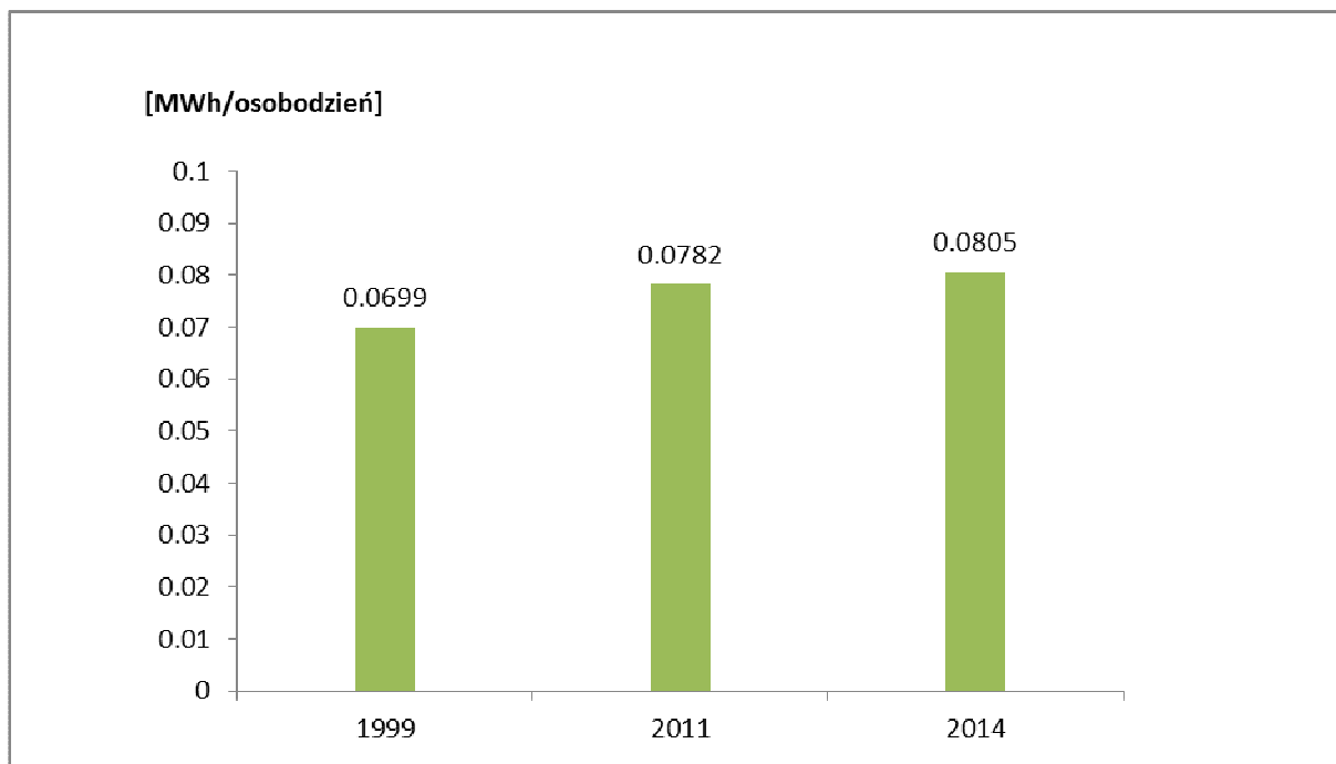
Rysunek 27. Zużycie energii na jeden osobodzień (mieszkańcy oraz turyści) z pominięciem przemysłu.
